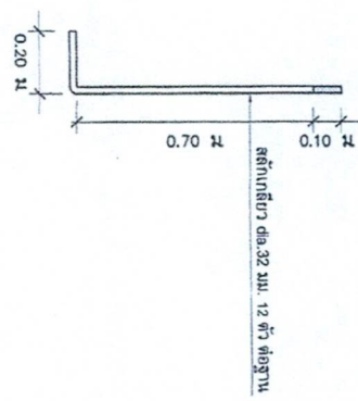
แบบขยายสลักเกลียวฐาน มาตราส่วน NO
